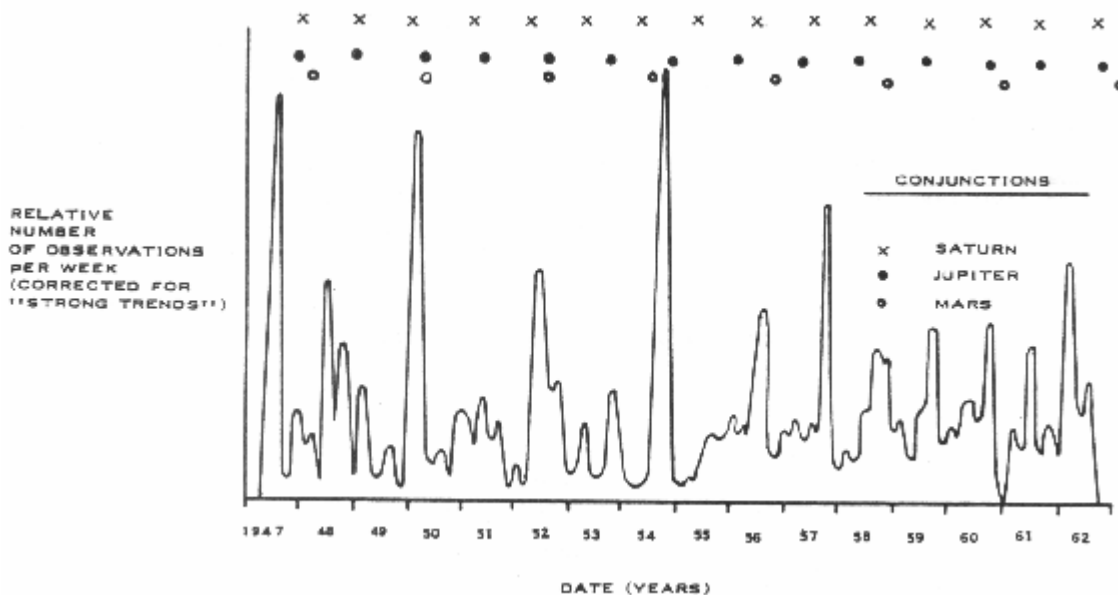
Abb. 33-2: Zyklen von Aktivität, mathematisch korrigiert auf "Starke Trends"
