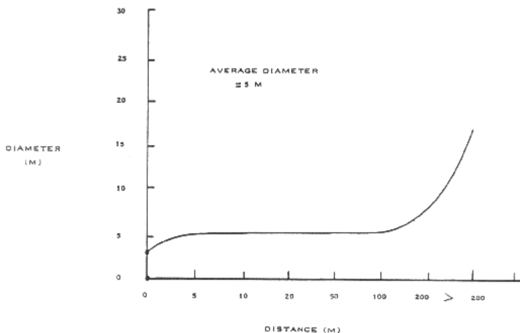
Abb. 33-1: UFO: Geschätzter Durchmesser [Diameter] in Relation zu der geschätzten Entfernung [Distance] vom Beobachter für UFOs unterhalb Baumwipfelhöhe
